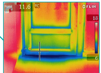
Défaut d'étanchéité La température de la porte au point (centre de la croix) est de 11,6°C. Les points faibles (infiltrations d'air) sont à 6°C.
