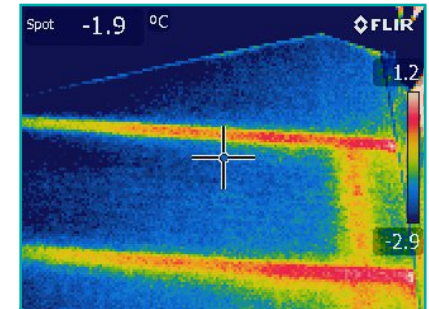
Ponts thermiques de dalles intermédiaires et mur de refend La température du mur au point (centre de la croix) est de -1,9°C. Les points faibles (ponts thermiques) sont à 1°C.
