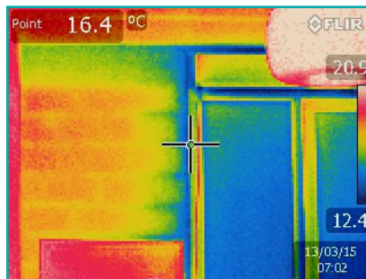
Défaut d'étanchéité La température de la menuiserie au point (centre de la croix) est de 16,4°C. Les points faibles (infiltrations d'air) sont à 12,4°C.
