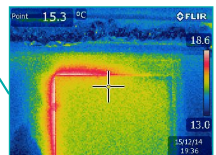
Défaut d'étanchéité La température de la porte au point (centre de la croix) est de 15,3°C. Les points faibles (infiltrations d'air) sont à 18,6°C.
