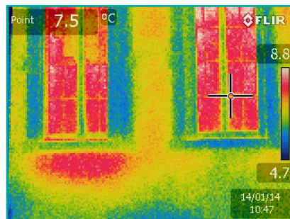
Radiateur sur mur extérieur non isolé La température extérieure du mur au niveau du radiateur est à 8°C, alors que le reste du mur est à environ 6°C.
