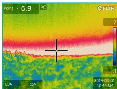
Pont thermique de plancher bas La température de la dalle (pont thermique) est de 6,9°C alors que le reste du mur est à 4°C.
