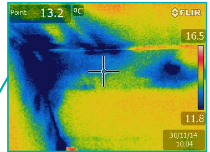
Tassement et infiltrations d'eau La température du plafond au point (centre de la croix) est de 13,2°C. Les points faibles (ponts thermiques) sont à 11,8°C.
