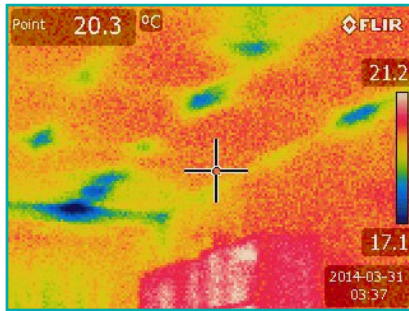
Ponts thermiques dus à une condensation aux liaisons de l'isolant La température du plafond au point (centre de la croix) est de 20,3°C. Les points faibles (ponts thermiques) sont à 17°C.
