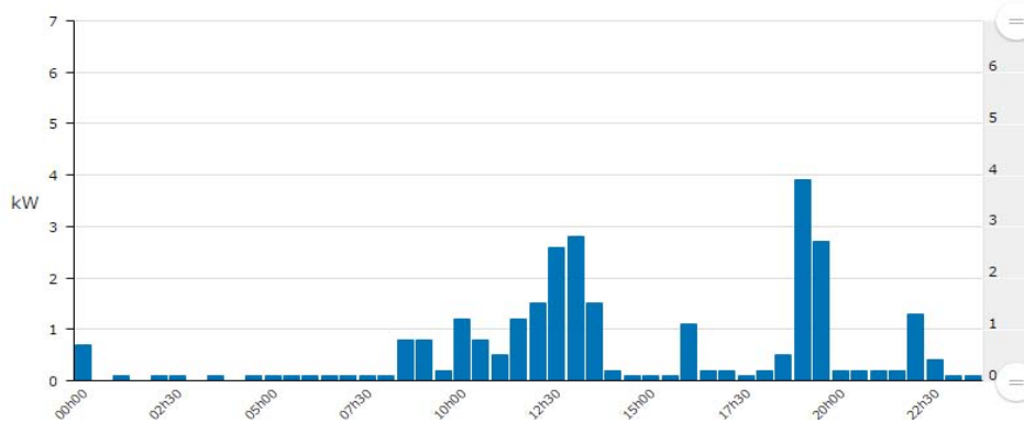
Courbes de puissance journalières appellées (courbe de charge en kW)
